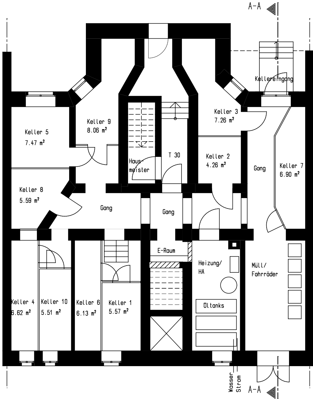
Kellergeschoss M 1:100
