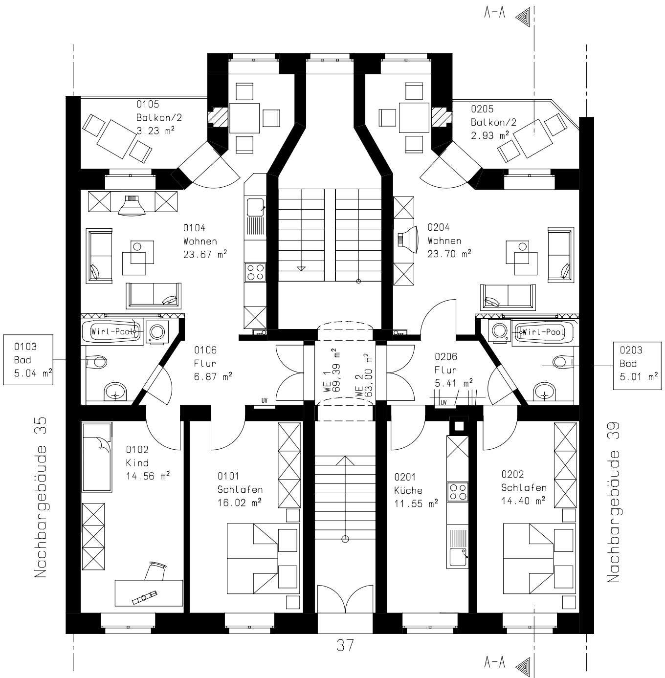
Erdgeschoss M 1:100
