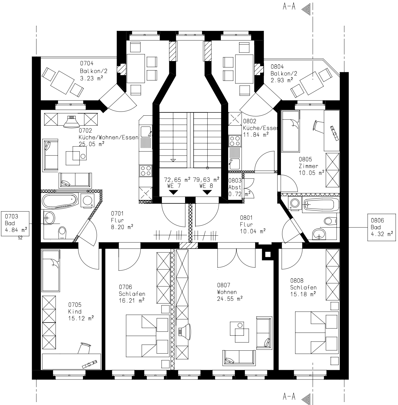
3. Obergeschoss M 1:100
